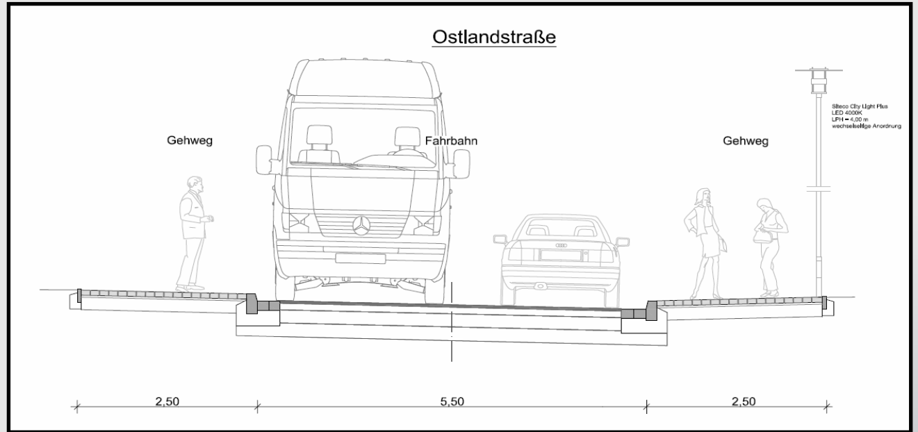
Regelprofil
