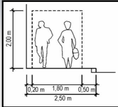
Straßenbegleitende Gehwege Regelbreite Seitenraum gem. RAS 06
